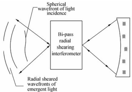
图 3 双通径向剪切干涉原理
