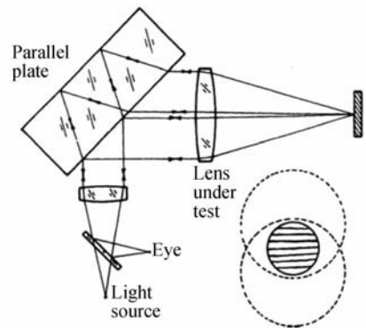
(b) Jamin 径向剪切干涉仪
