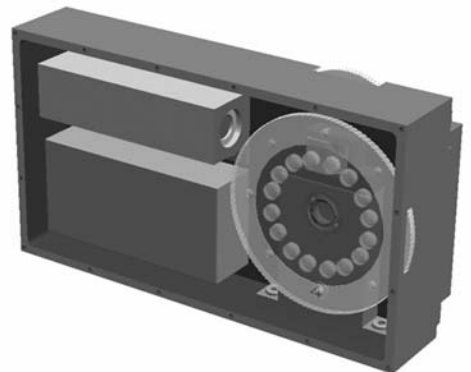
图 4 剪切干涉仪光机系统设计实例
