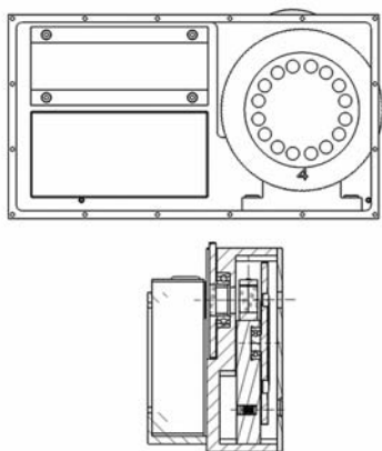
图5 剪切干涉仪结构设计
